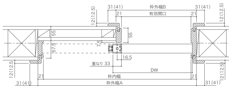
横断面図
