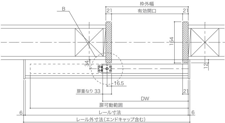
固定枠仕様
