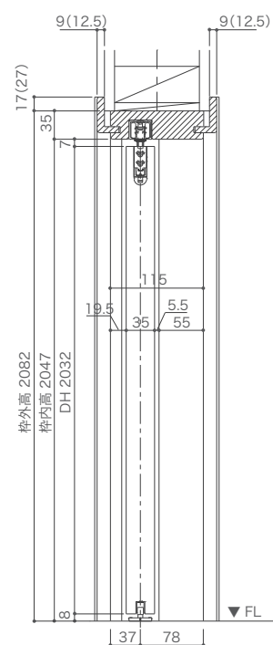
縦断面図
