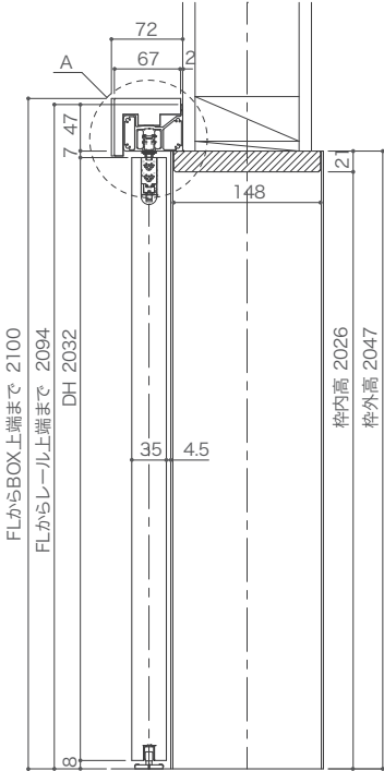
縦断面図
