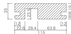
上枠
