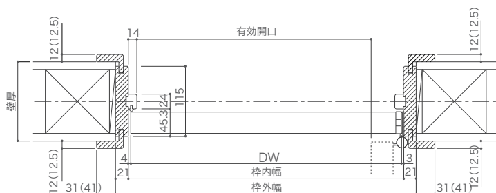
横断面図
