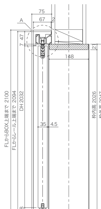
縦断面図
