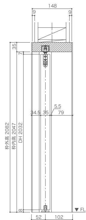
縦断面図
