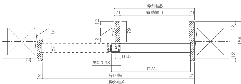
横断面図
