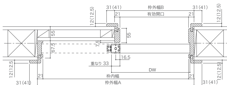
横断面図
