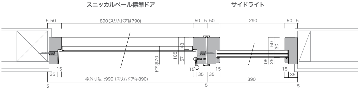
横断面図
