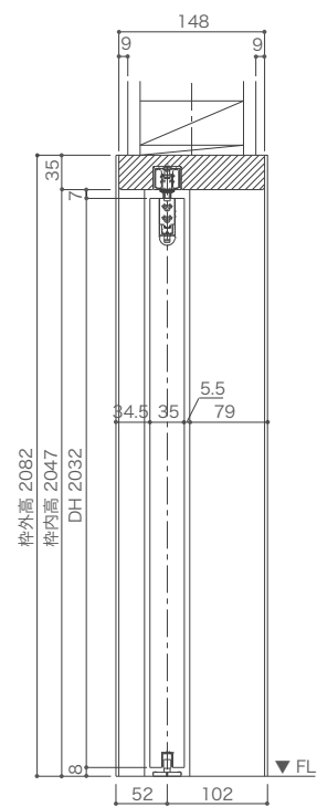
縦断面図
