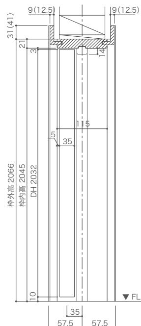
縦断面図
