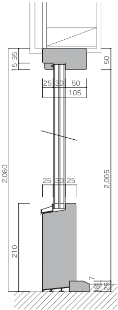
縦断面図
