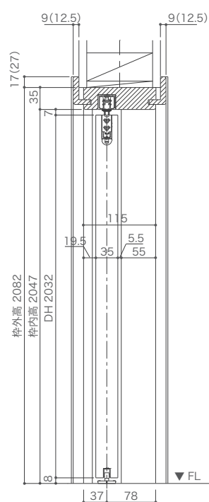
縦断面図
