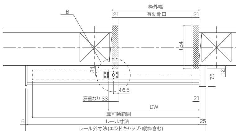
横断面図
