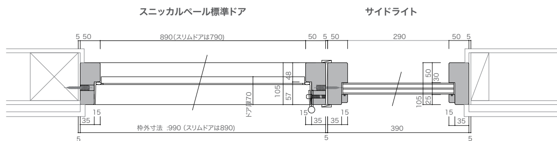
横断面図
