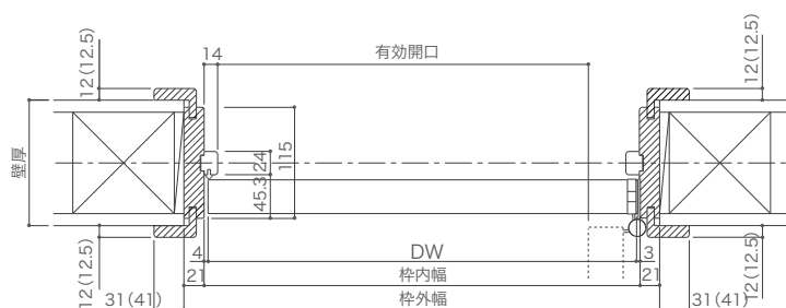
横断面図
