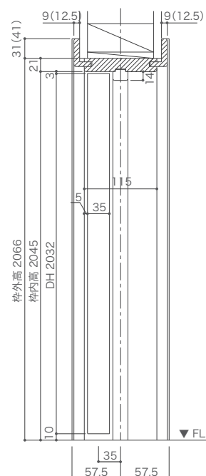
縦断面図
