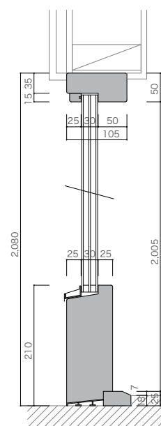
縦断面図
