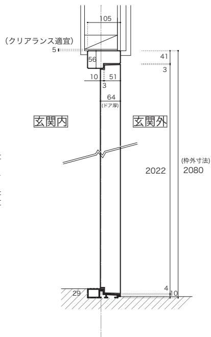
縦断面図
