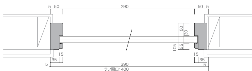
横断面図
