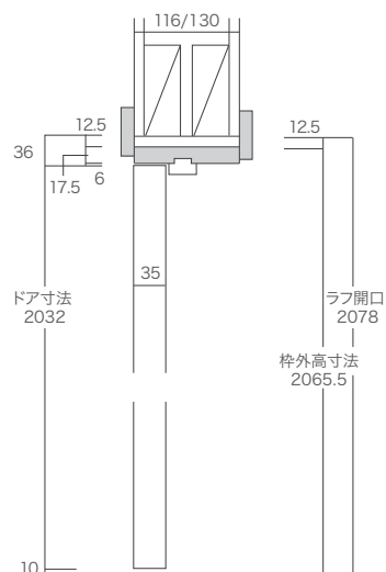
縦断面図
