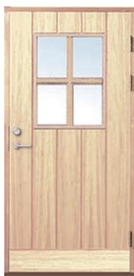
YD251G パイン ¥650,000 熱貫流率 1.05w/㎡・K ◎型トリプルガラス
