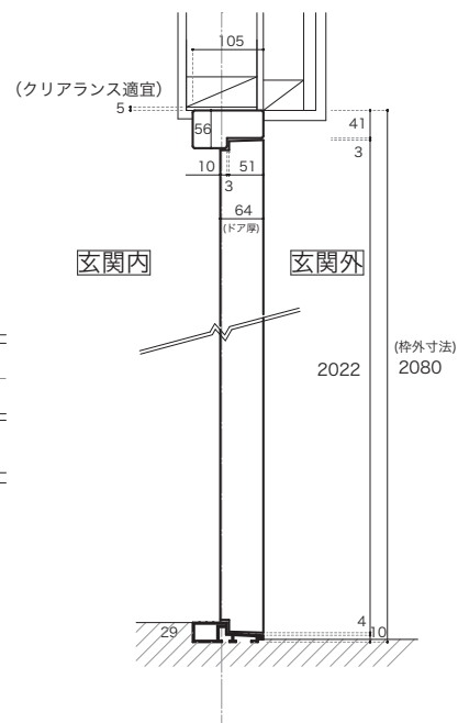
縦断面図
