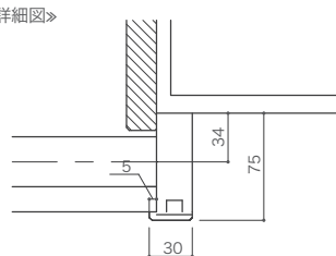
《縦枠部分詳細図》
