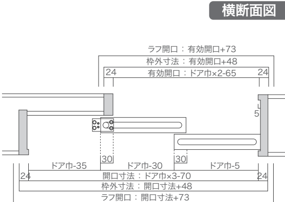
連動2本引き込み戸標準納まり図
