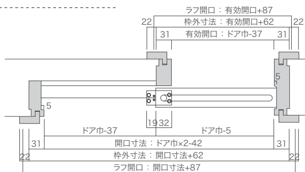
引違い横断面図
