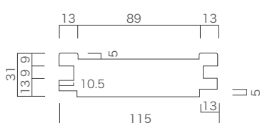
縦枠 (引違い用)
