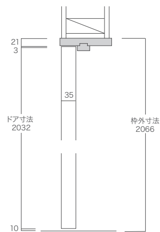
縦断面図
