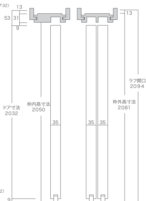
縦断面図
