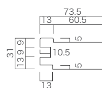
戸当たり
