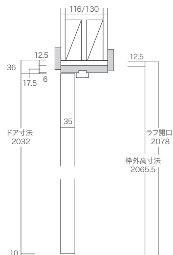
縦断面図
