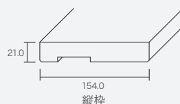
縦枠
