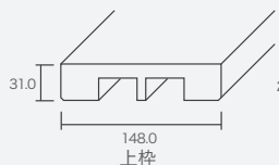
上枠
