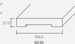
縦枠
