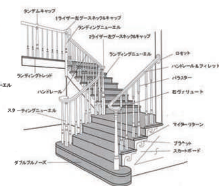
OVER THE POST オーバー・ザ・ポスト
