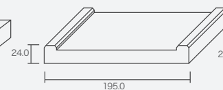
3本引き込み戸用 縦枠
