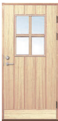
YD251G パイン ¥620,000 熱貫流率 1.05w/㎡・K ◎型トリプルガラス
