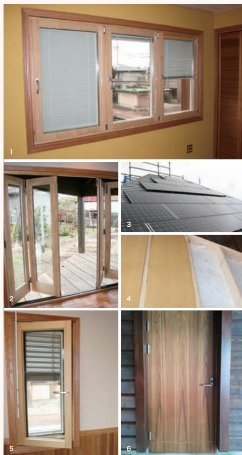
1 超高性能木製窓 内蔵ブラインド 2 アンダーセン・ファールディングドア 3 太陽光発電による創エネエネルギー 4 断熱材の強化 5 超高性能木製窓 外部ブラインド 6 玄関ドア（MD251チーク）
