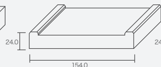
2本引き込み戸用 縦枠
