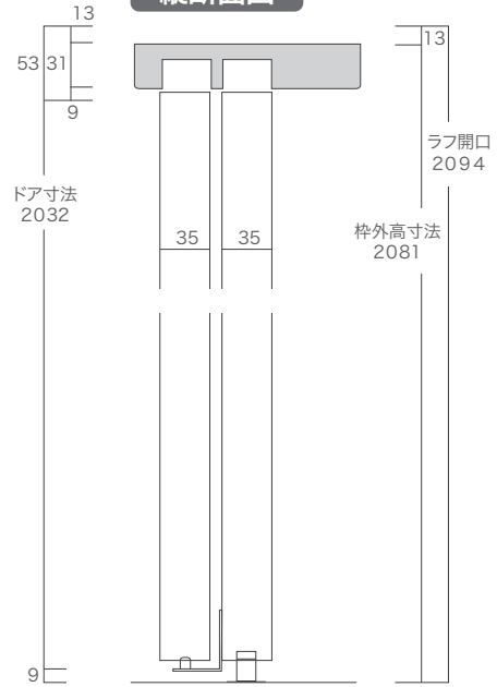
縦断面図
