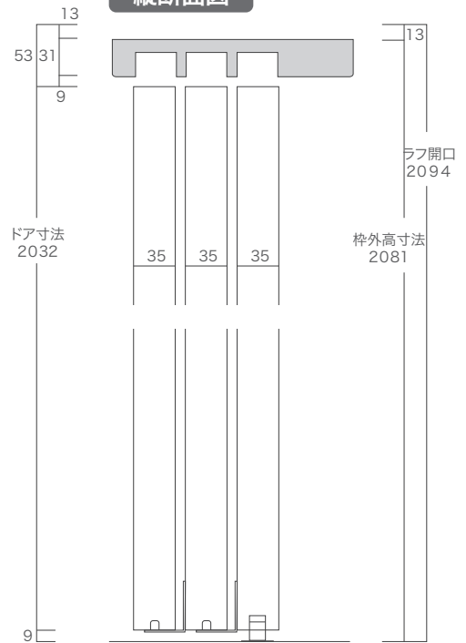
縦断面図
