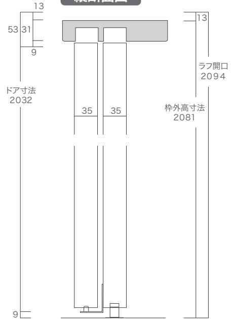
縦断面図
