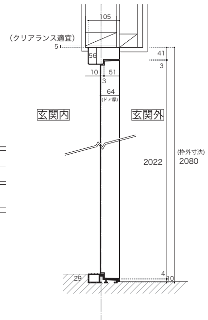
縦断面図
