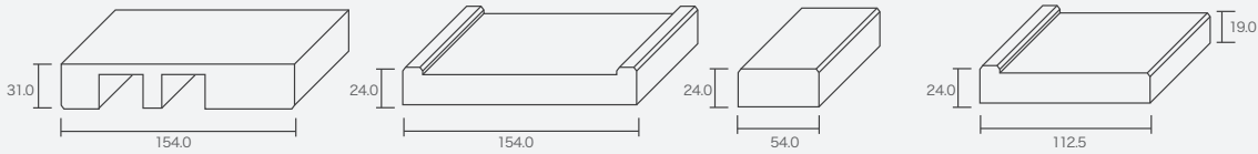
2本引き込み戸用 上部枠
