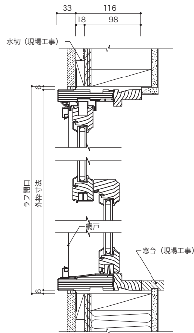
垂直断面図
