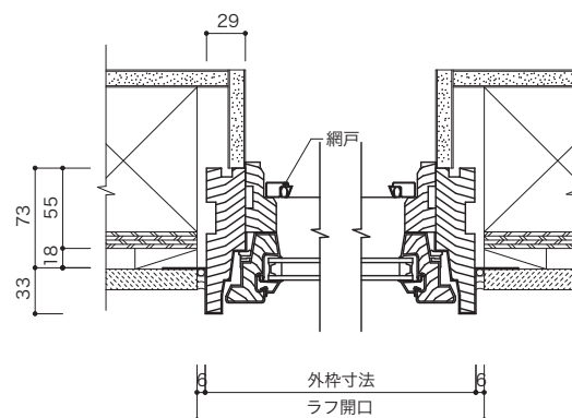
水平断面図
