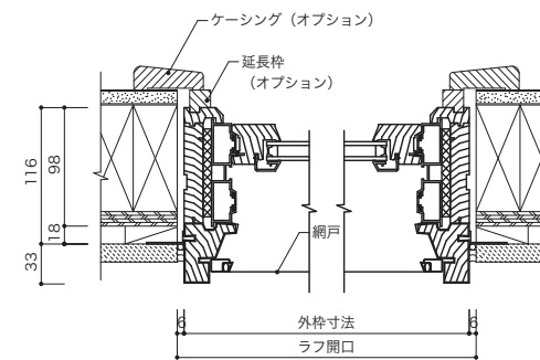
垂直断面図
