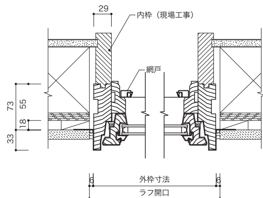
水平断面図
