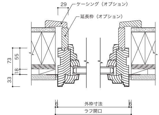
垂直断面図
