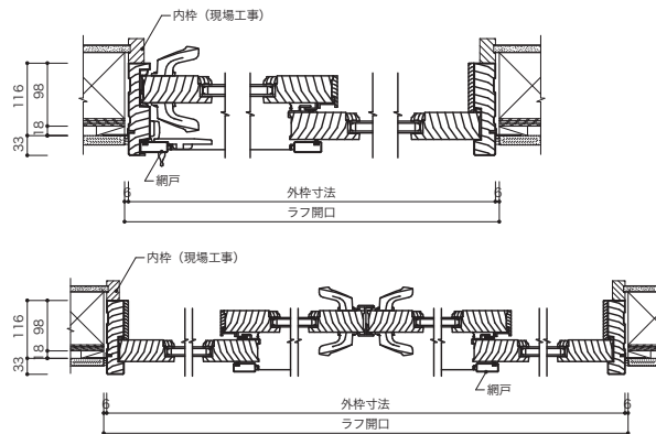
水平断面図
