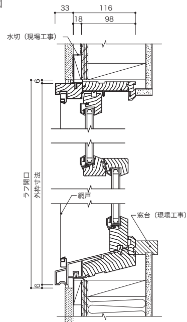
垂直断面図
