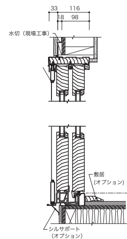
垂直断面図
