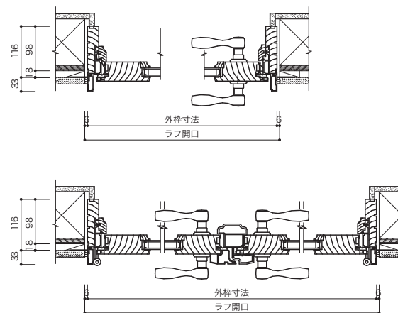
垂直断面図
