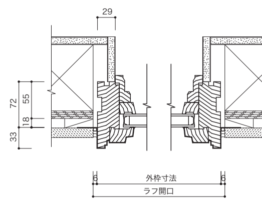
垂直断面図
