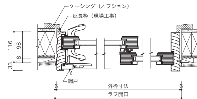
水平断面図
