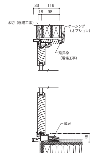
垂直断面図
