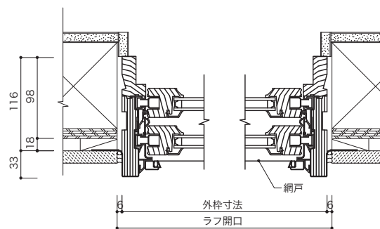
垂直断面図
