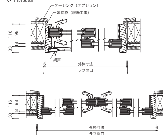
水平断面図
