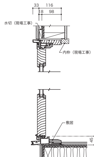
垂直断面図
