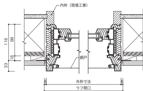
垂直断面図
