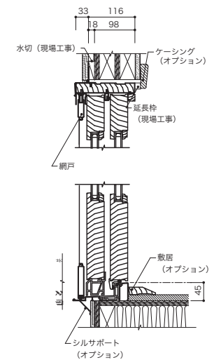
垂直断面図
