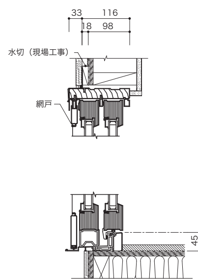
垂直断面図
