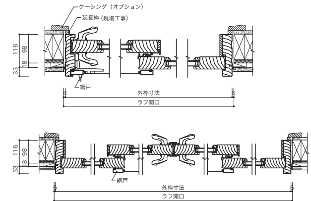
水平断面図
