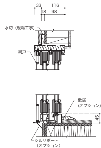
垂直断面図
