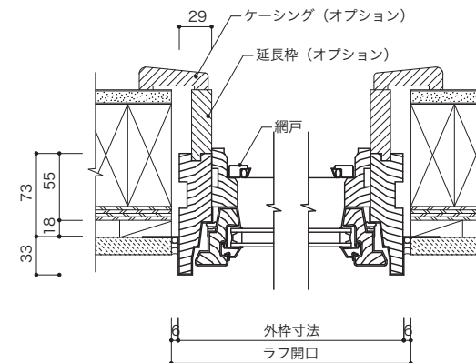
水平断面図
