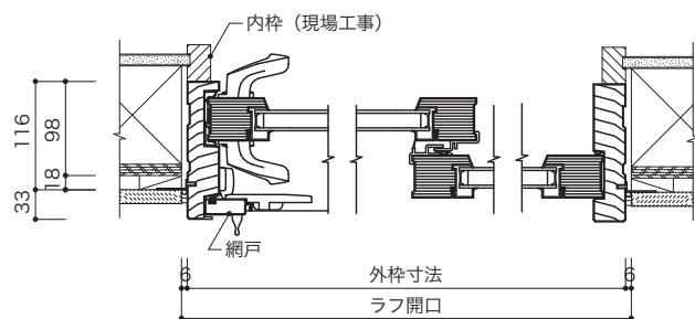
水平断面図
