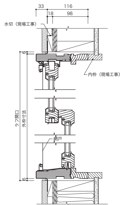
垂直断面図
