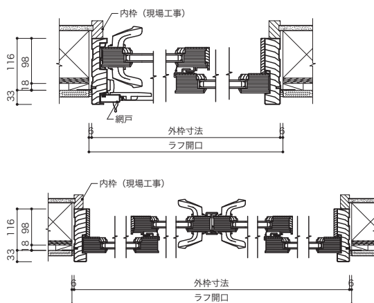
水平断面図
