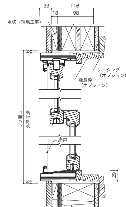
垂直断面図
