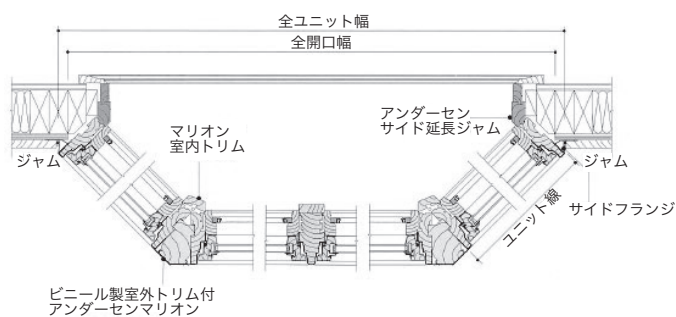
水平断面図
