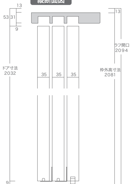
縦断面図
