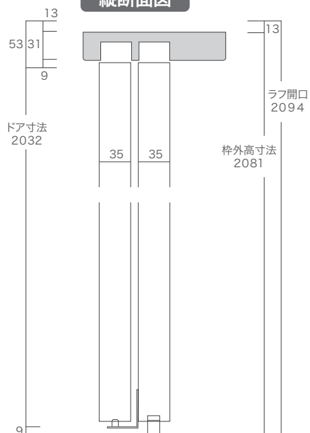
縦断面図
