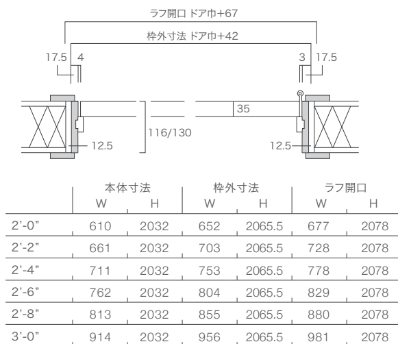
横断面図
