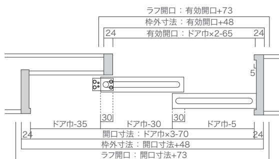
横断面図
