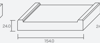
2本引き込み戸用 縦枠
