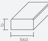
3本引き込み戸用 方立
