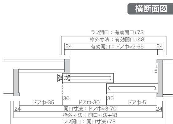
連動 2 本引き込み戸標準納まり図
