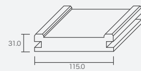
引き戸用 縦枠 (左右兼用)
