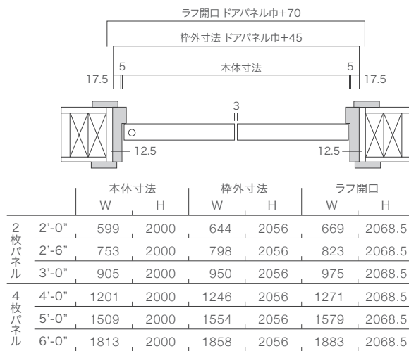
横断面図
