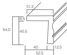
357型ケーシング 40
