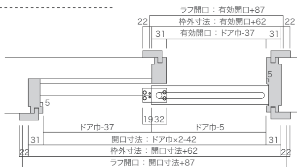
引戸標準納まり図 (差込枠)
