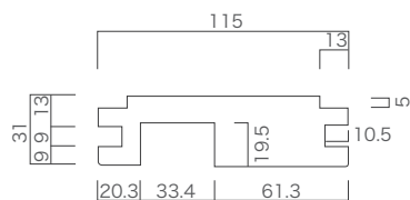
上枠 (片引き用)
