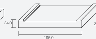
3本引き込み戸用 縦枠
