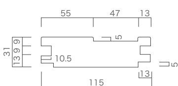
縦枠 (片引き用)
