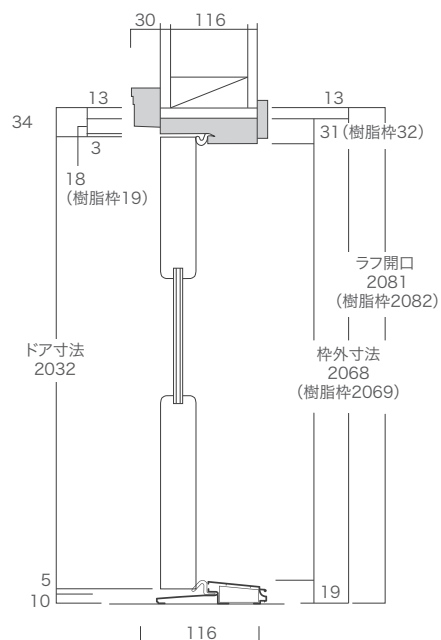
縦断面図
