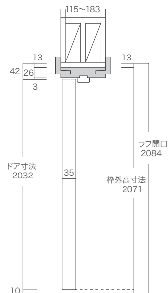
縦断面図
