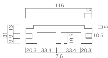
縦枠 (引違い用)
