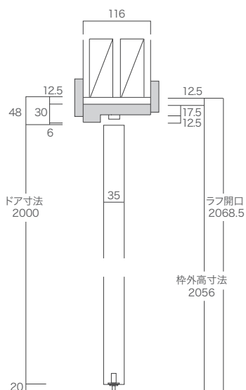
縦断面図
