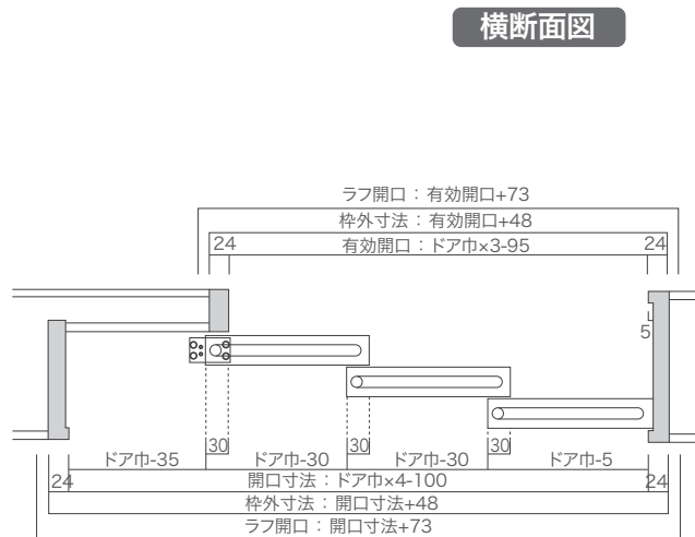
連動 3 本引き込み戸標準納まり図
