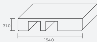
2本引き込み戸用 上部枠
