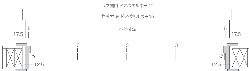
横断面図
