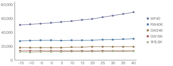
各種断熱材の熱容量の値は、樹木の繊維で実施した比熱測定結果より算出（比熱×密度＝熱容量） 比熱測定：株式会社 アグネ技術センターにて「真空理工製比熱測定装置 SH-3000 型」を使用し測定 ※羊毛断熱材の密度（8kg/ m³）は樹木の繊維での実測値 資料：株式会社木の繊維
