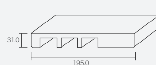
3本引き込み戸用 上部枠
