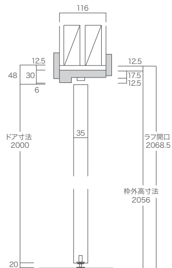
縦断面図
