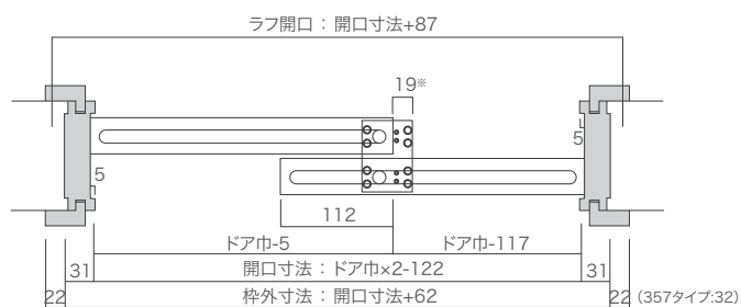
引違い横断面図
