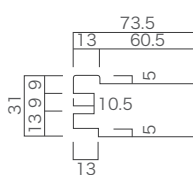
戸当り
