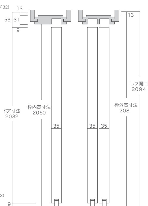
縦断面図
