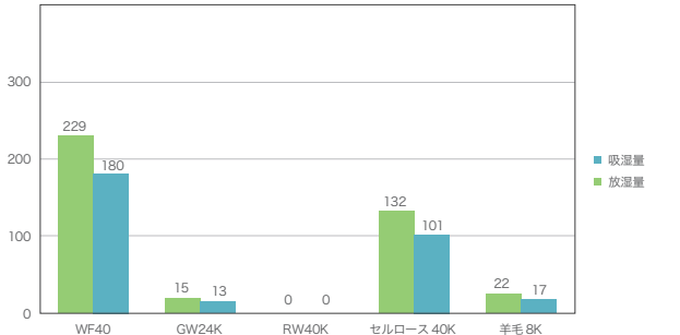
一般財団法人 建材試験センターにて JIS A 6901（せっこうボード製品）の 7.14 吸放湿性試験に準じて行った試験結果による（試験条件：寸法 250mm×250mm×50mm厚、乾燥 50℃、養生 23℃53%RH、吸湿過程 24 時間 23℃93%RH、放湿過程 24 時間 23℃53%RH）資料：株式会社木の繊維
