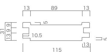
縦枠 (引違い用)
