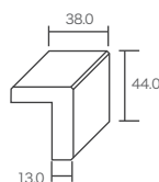
L型ケーシング 25
