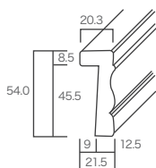
357型ケーシング 09
