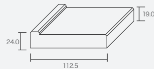
2本引き込み戸用 戸当
