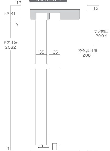
縦断面図
