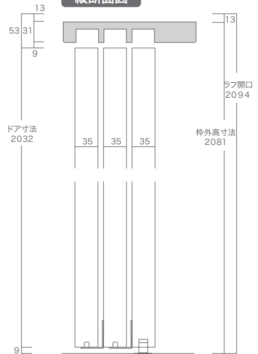
縦断面図
