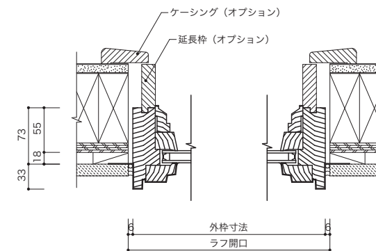
垂直断面図
