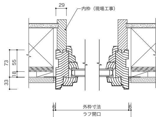
垂直断面図
