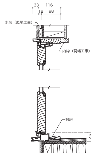
垂直断面図
