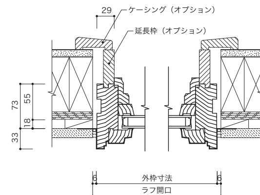
垂直断面図
