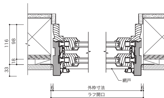
垂直断面図
