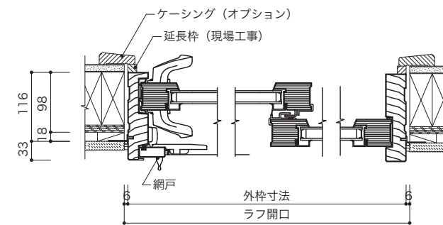
水平断面図
