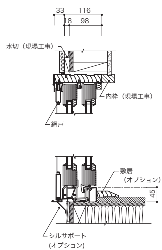
垂直断面図
