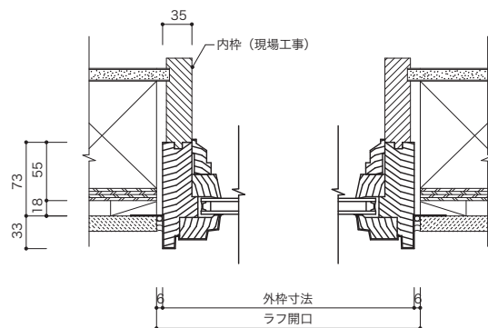
垂直断面図
