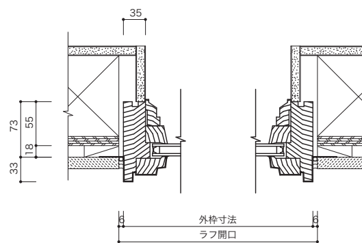
垂直断面図
