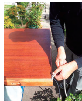
④コーキング、タッカーをカッターやヘラで除去します。
