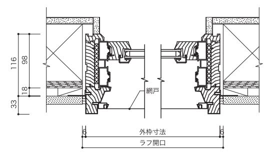
垂直断面図
