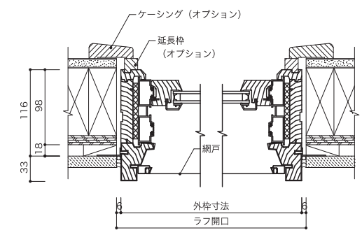
垂直断面図
