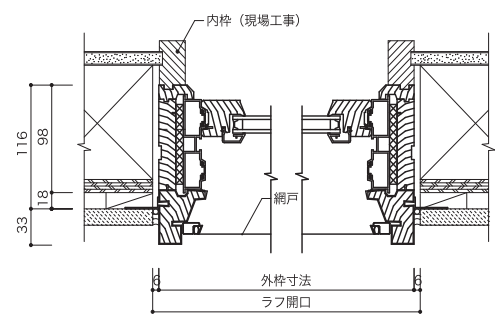
垂直断面図
