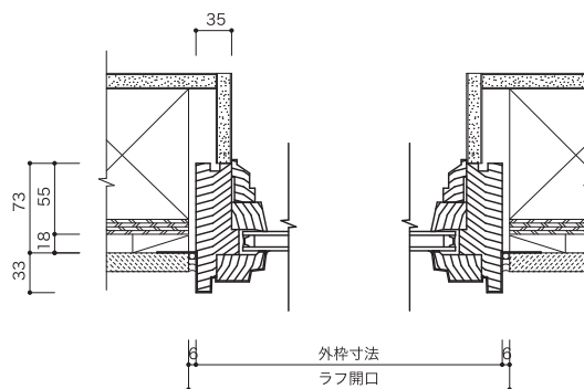
垂直断面図
