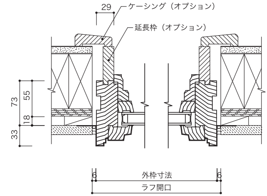
垂直断面図
