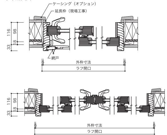
水平断面図
