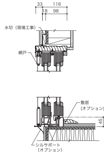
垂直断面図
