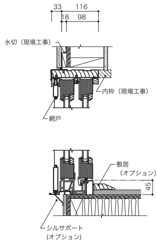
垂直断面図
