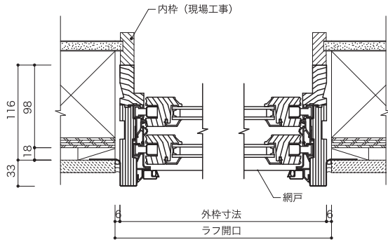
水平断面図
