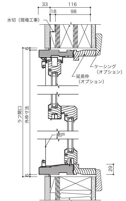
垂直断面図
