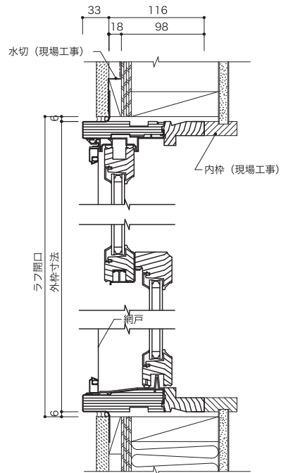
垂直断面図
