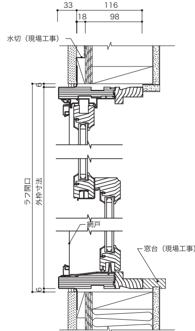
垂直断面図
