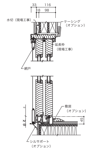
垂直断面図
