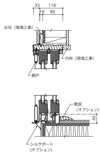
垂直断面図
