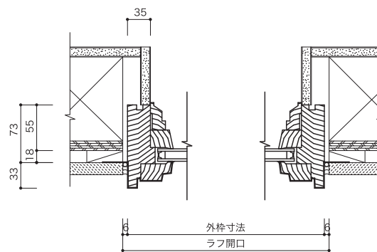
垂直断面図
