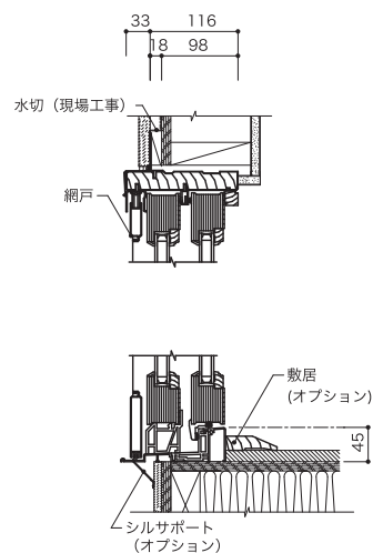
垂直断面図
