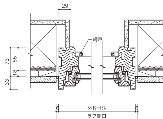
水平断面図
