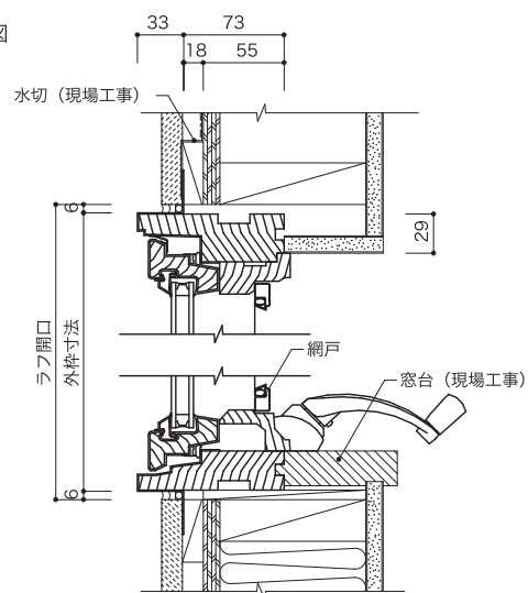
垂直断面図
