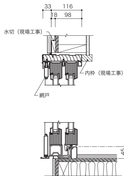
垂直断面図
