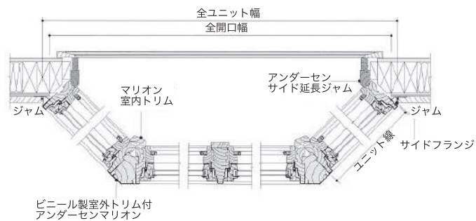
水平断面図
