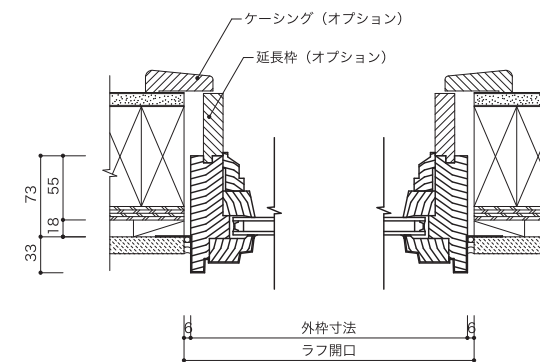
垂直断面図
