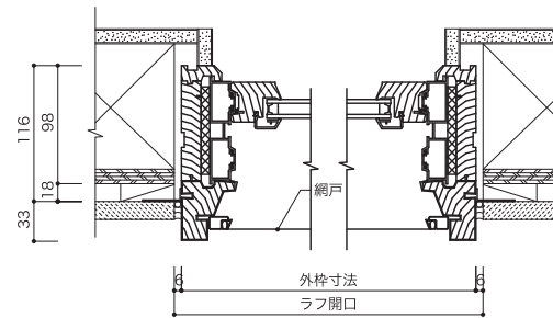
垂直断面図
