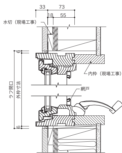
垂直断面図
