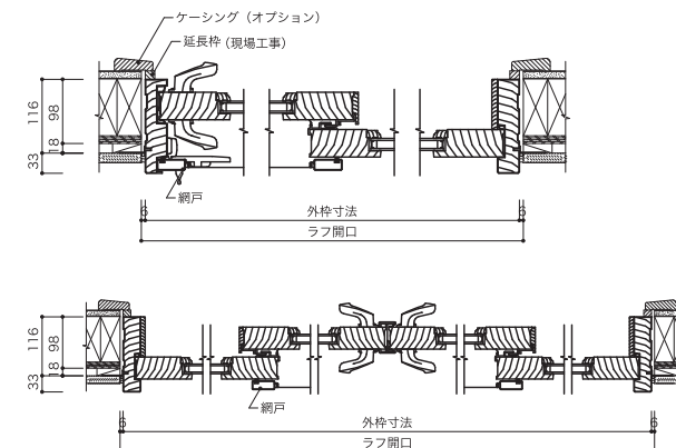
水平断面図
