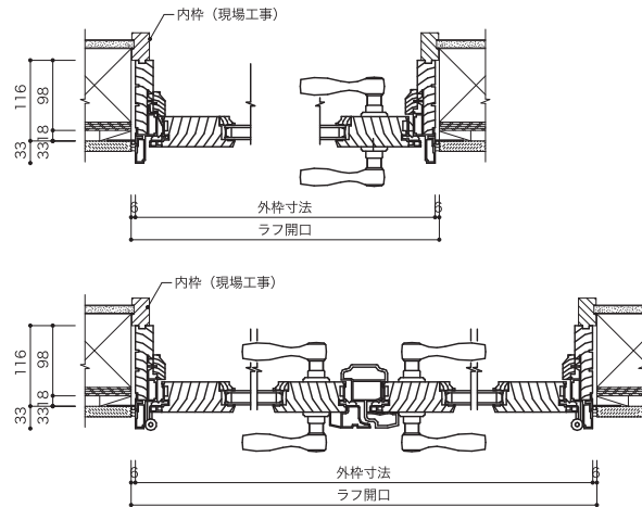
水平断面図
