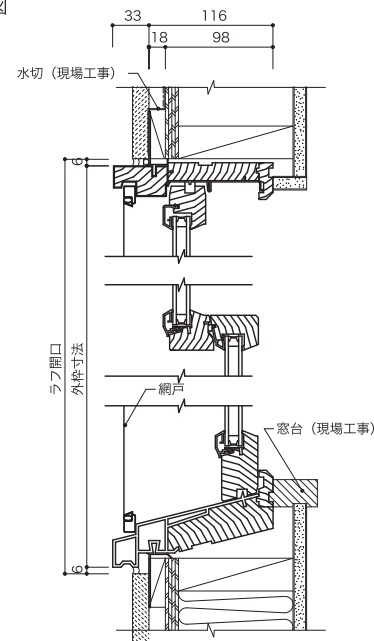
垂直断面図
