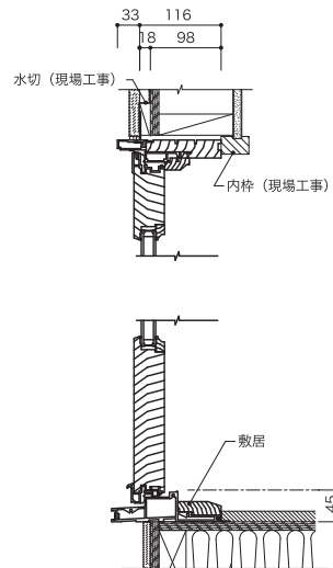
垂直断面図
