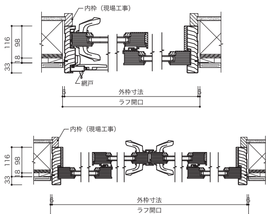
水平断面図
