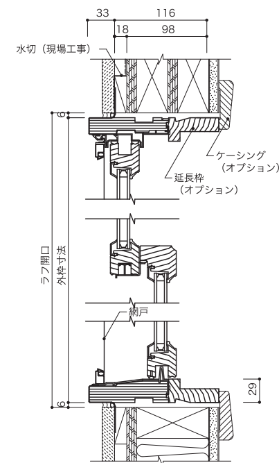
垂直断面図
