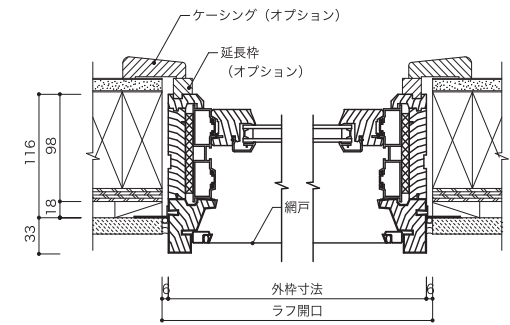
垂直断面図
