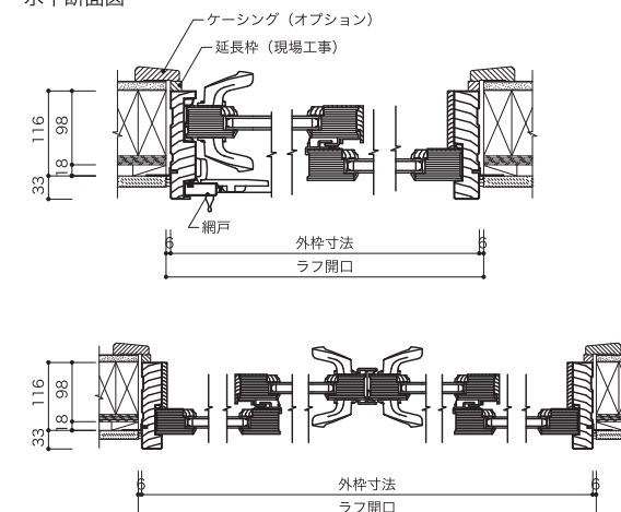
水平断面図
