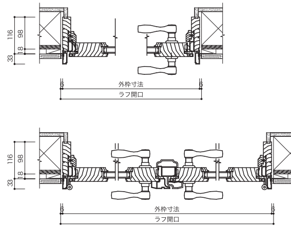
垂直断面図
