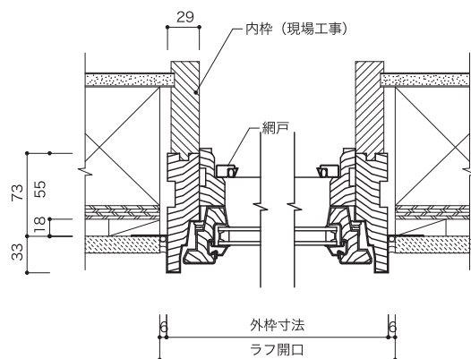
水平断面図
