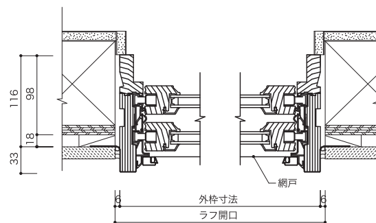
垂直断面図
