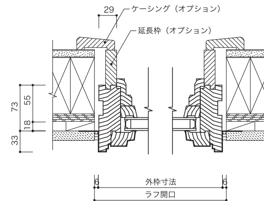
垂直断面図
