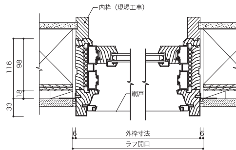
垂直断面図
