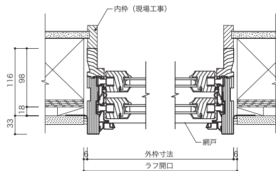
水平断面図
