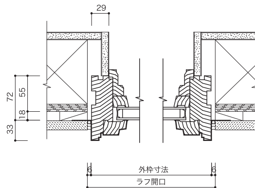
垂直断面図
