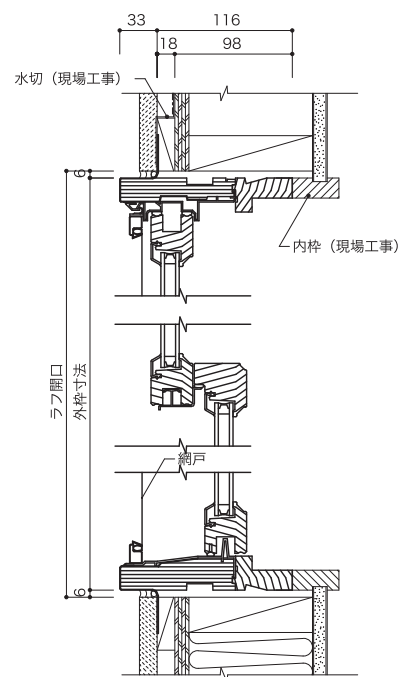
垂直断面図
