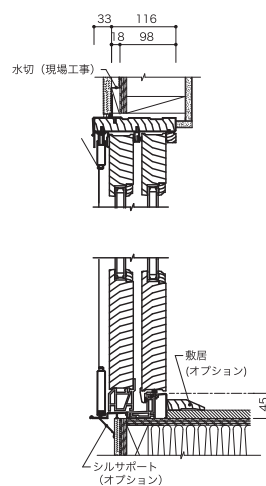
垂直断面図
