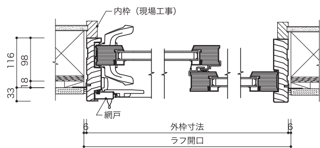
水平断面図
