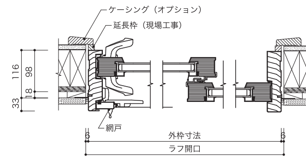
水平断面図
