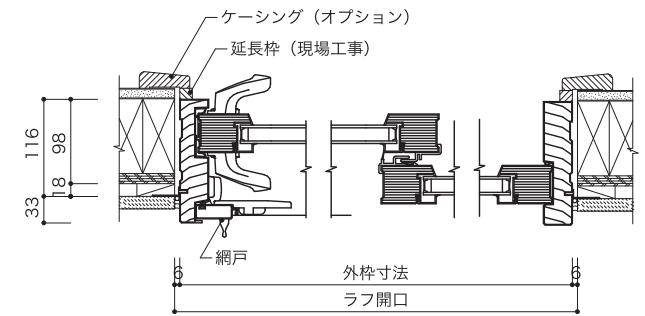
水平断面図
