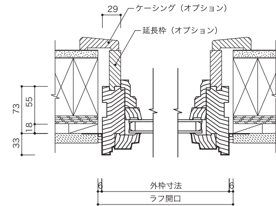
垂直断面図
