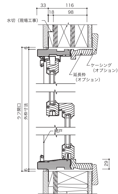
垂直断面図
