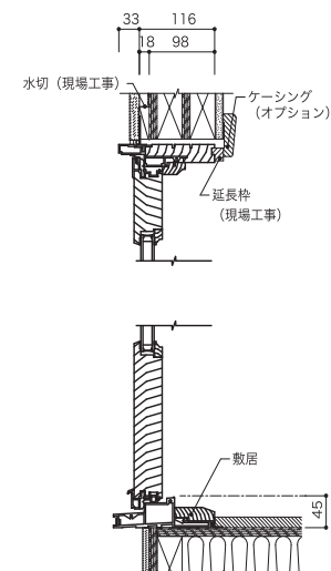
垂直断面図
