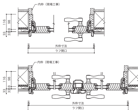
水平断面図
