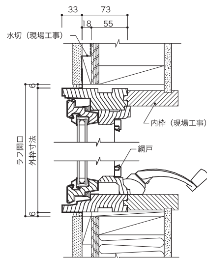
垂直断面図
