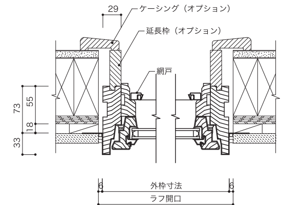
水平断面図
