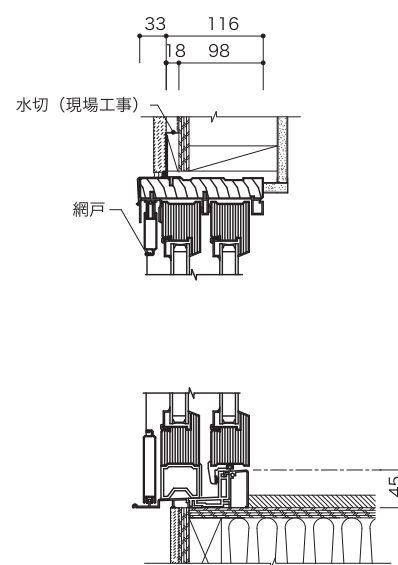
垂直断面図
