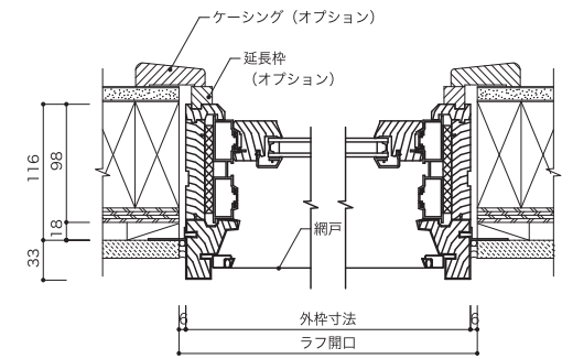
垂直断面図
