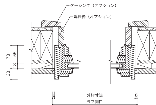
垂直断面図
