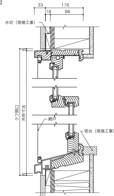
垂直断面図
