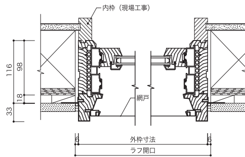
垂直断面図
