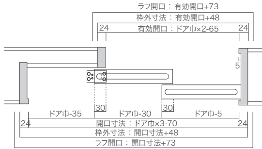
横断面図
