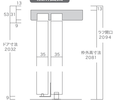
縦断面図
