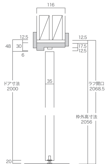
縦断面図
