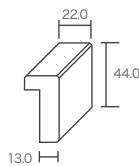
L型ケーシング 09 ℓ = 3' -965 mm ¥1,200 ℓ = 7' -2133 mm ¥2,400 壁厚 115~124 mm 対応
