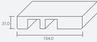
2本引き込み戸用 上部枠 ℓ = 2682 mm
