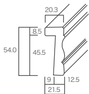
357型ケーシング 09 ℓ = 965 mm ¥1,900 ℓ = 7' -2133 mm ¥3,800 壁厚 115~124 mm 対応
