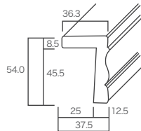
357型ケーシング 25 ℓ = 965 mm ¥1,900 ℓ = 7' -2133 mm ¥3,800 壁厚 115~153 mm 対応
