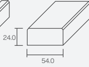
2本引き込み戸用 方立 ℓ = 2200 mm
