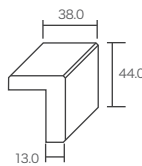
L型ケーシング 25 ℓ = 3' -965 mm ¥1,400 ℓ = 7' -2133 mm ¥2,800 壁厚 115~153 mm 対応
