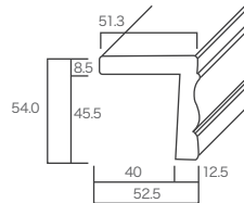
357型ケーシング 40 ℓ = 965 mm ¥2,200 ℓ = 7' -2133 mm ¥4,400 壁厚 143~183 mm 対応
