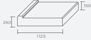
2本引き込み戸用 戸当 ℓ = 2200 mm
