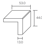
L型ケーシング 40 ℓ = 3' -965 mm ¥1,700 ℓ = 7' -2133 mm ¥3,400 壁厚 143~183 mm 対応
