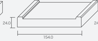
2本引き込み戸用 縦枠 ℓ = 2200 mm
