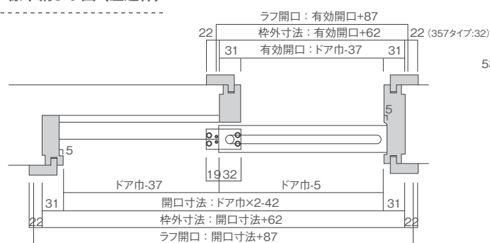
引戸標準納まり図 (差込枠)
