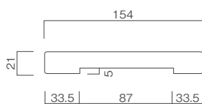
縦枠 (引違い戸)
