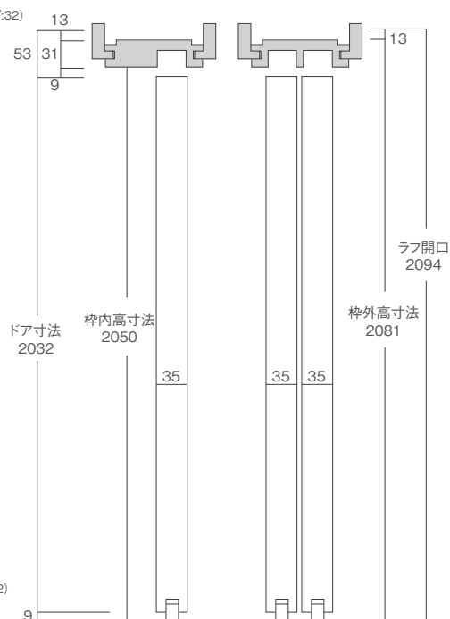
縦断面図
