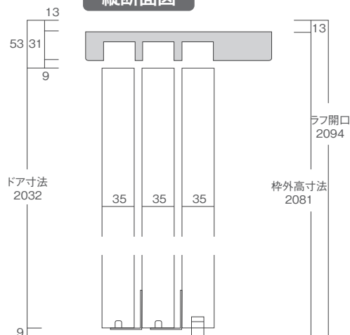
縦断面図
