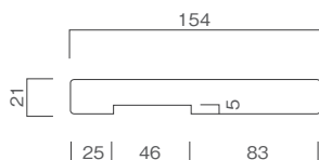
縦枠 (引違い戸)
