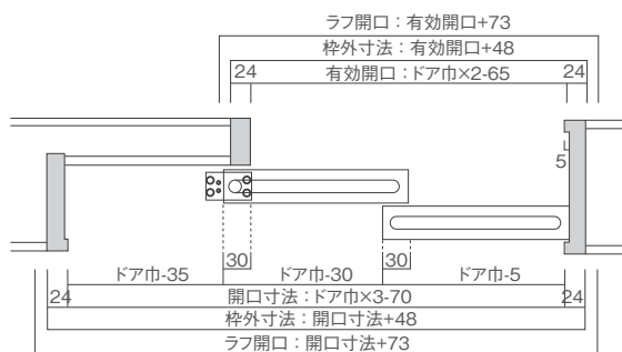
横断面図
