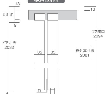
縦断面図
