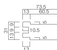
戸当り
