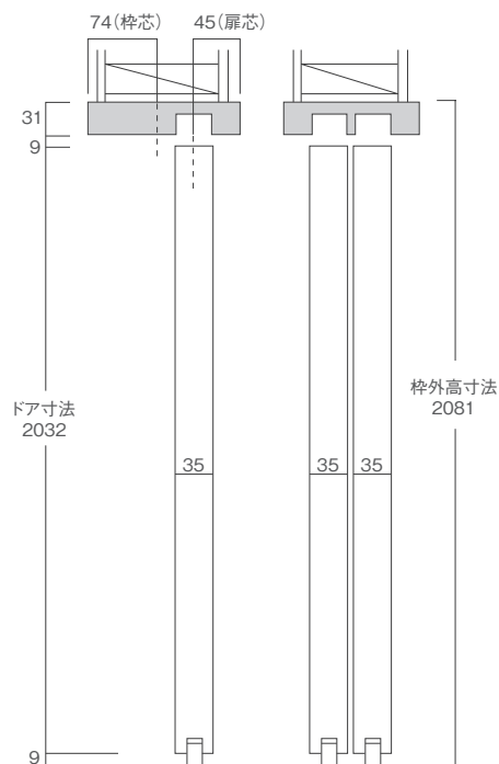
縦断面図
