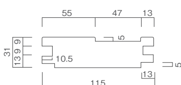
縦枠 (片引き用)
