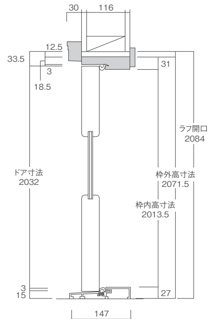
縦断面図
