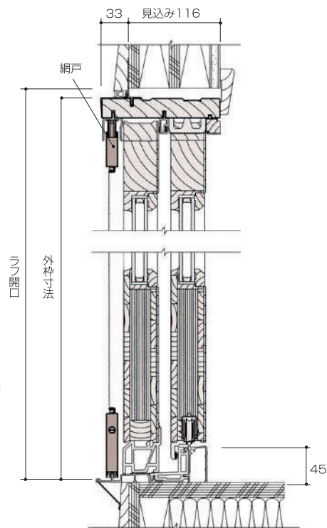
垂直断面図
