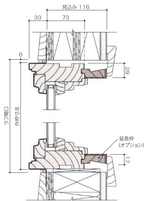
垂直断面図
