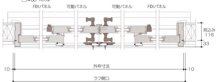
水平断面図
