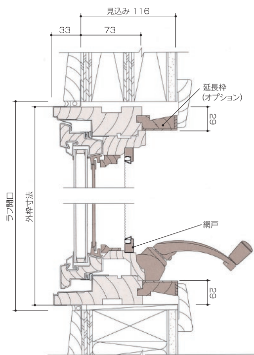
垂直断面図
