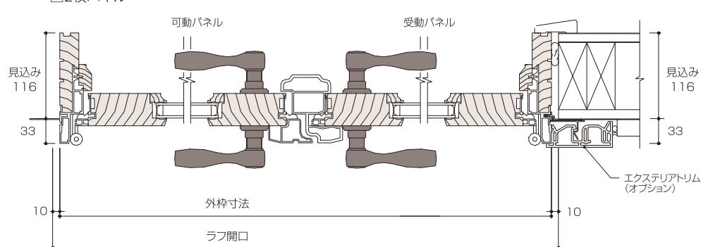
水平断面図
