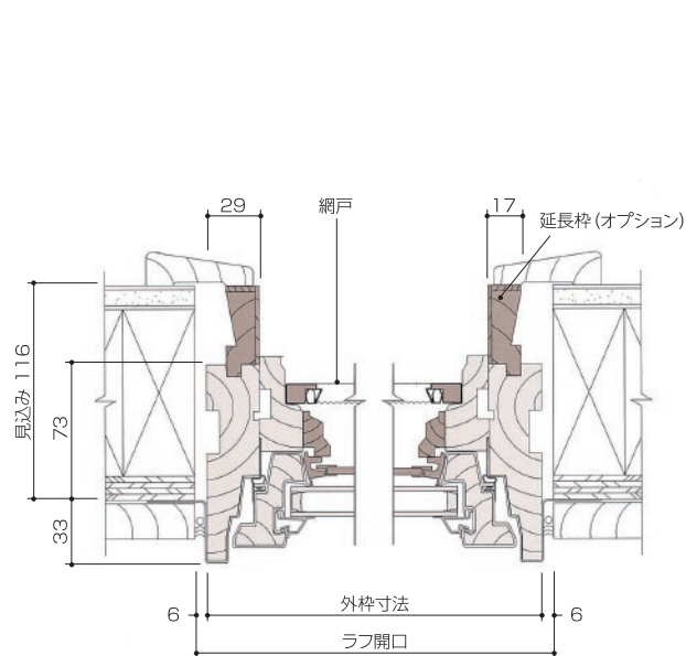
水平断面図
