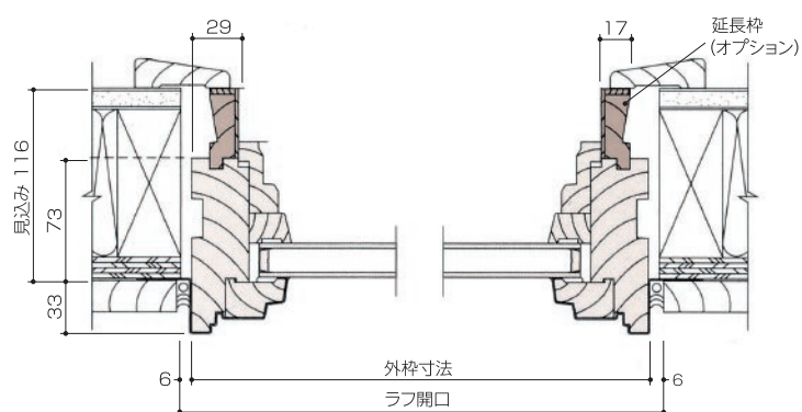
水平断面図
