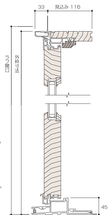
垂直断面図
