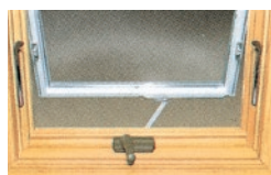
オーニングサッシロック 左右のコーナーロックにより防犯と気密性がさらに高まります。
